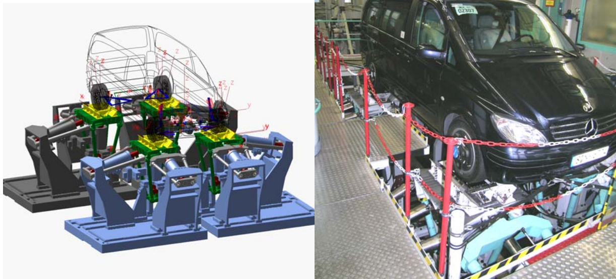
Bild 2: MKS-Modell und realer Prüfstand
