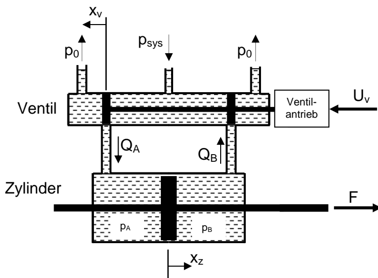
Bild 7: Modell des Servoventils und der Aktuatorik
