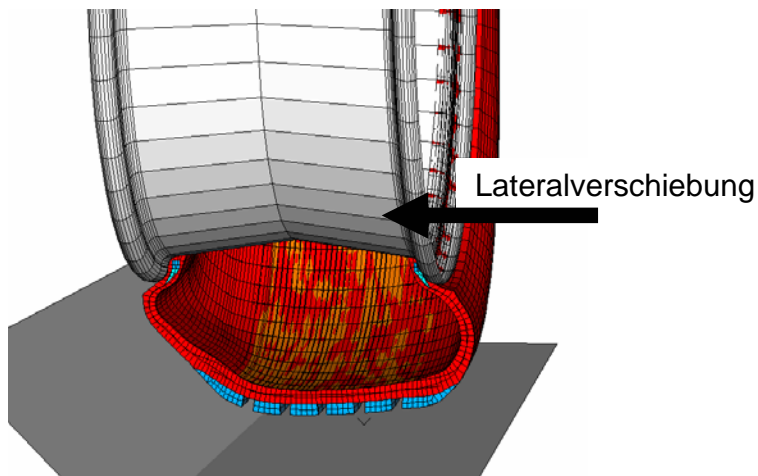
Bild 5: FE-Rechnung mit Kontakt (ABAQUS) zur Ermittlung der Lateralsteifigkeit
