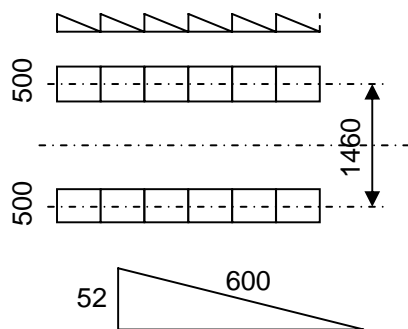
Bild 8: Hindernis Sägezahn
