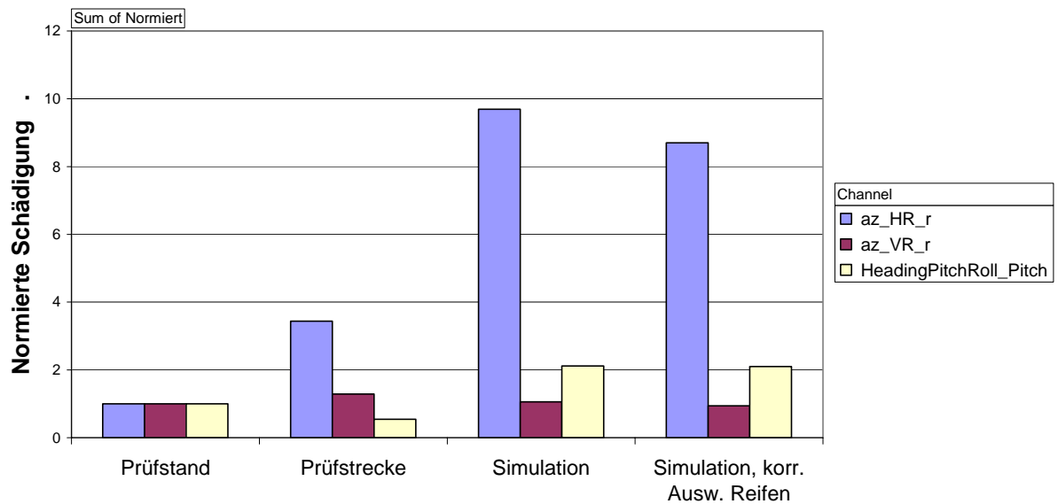
Bild 12: Schädigungsvergleich für Achsbeschleunigungen und Nickwinkel
