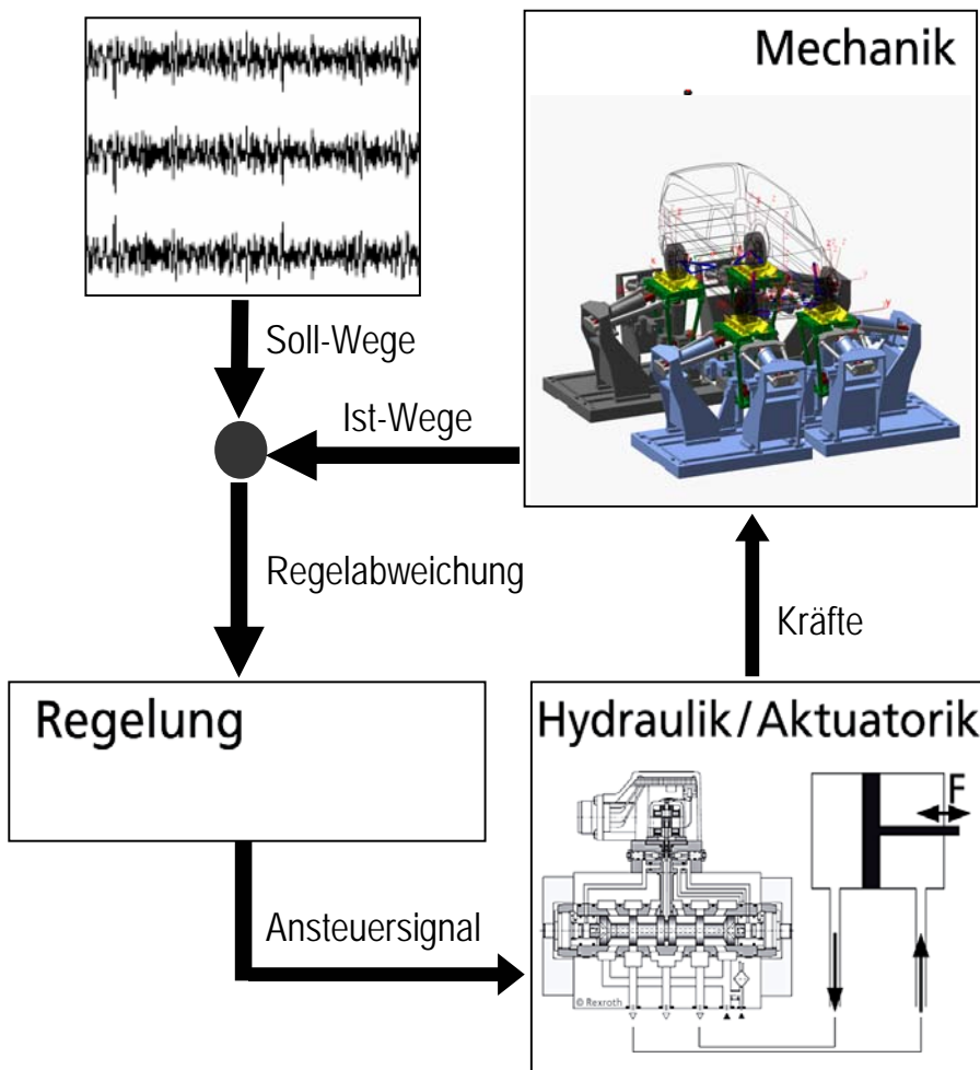
Bild 1: DaimlerChrysler ET/GF Transporter-Prüfstand: Gesamtsystem
