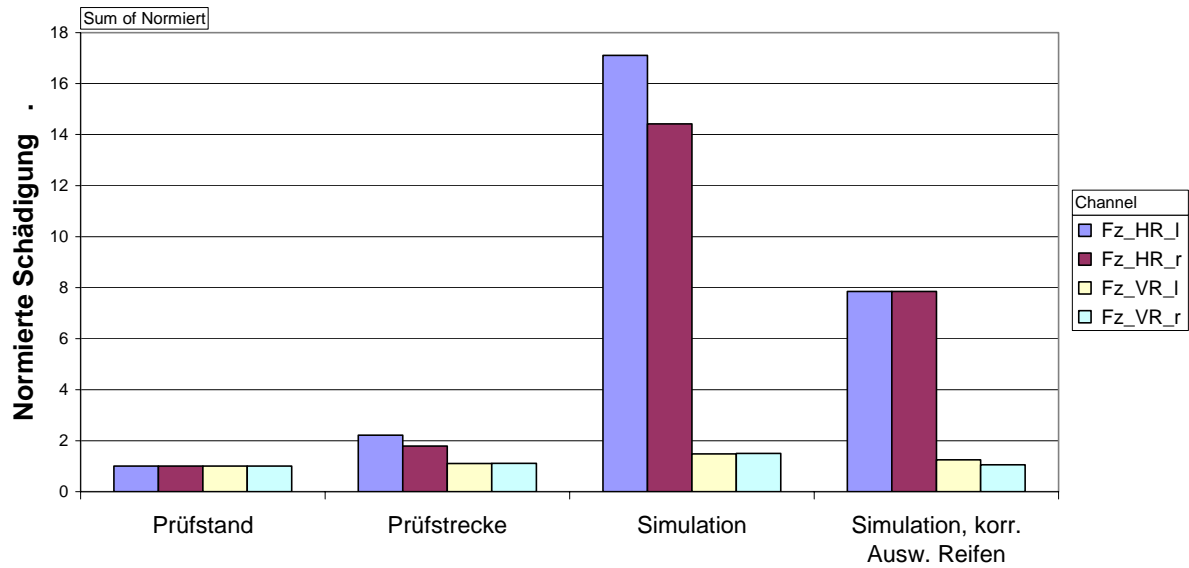
Bild 11: Schädigungsvergleich für Vertikalkräfte
