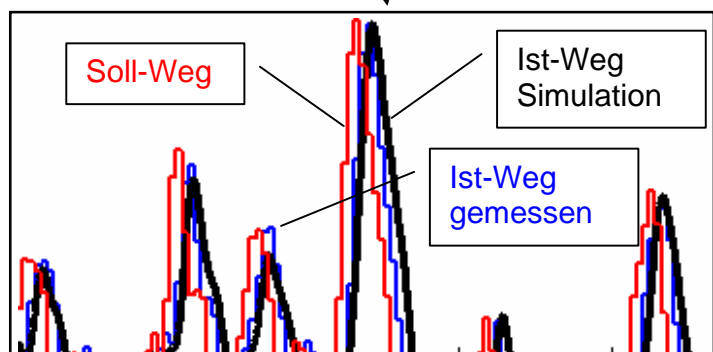
Bild 17: Vergleich Soll-Weg vertikal mit Ist-Weg gemessen am Prüfstand und aus Simulation (für Rauschsignal)
