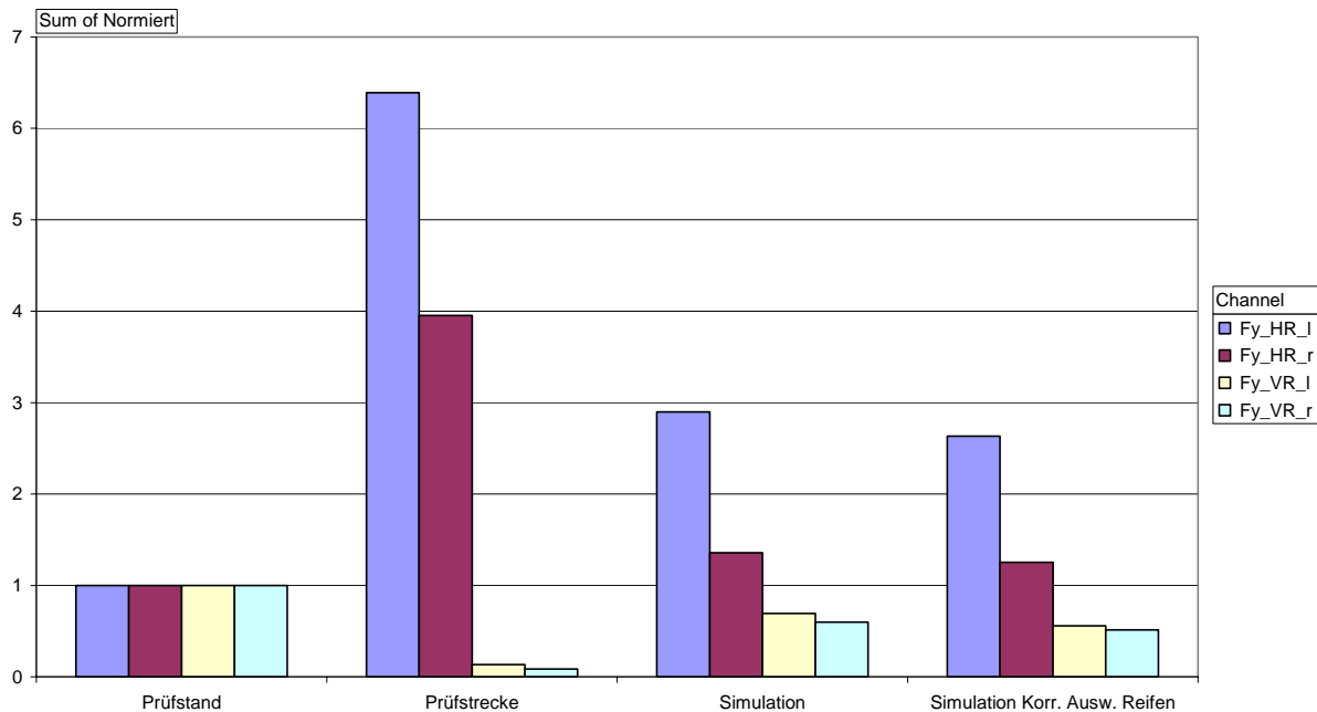
Bild 13: Schädigungsvergleich für Lateralkräfte
