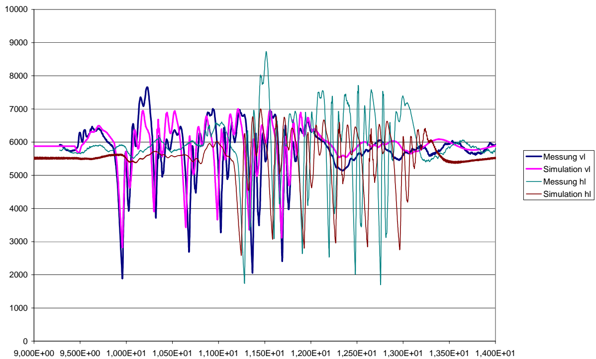
Bild 9: Vergleich Messung zu Simulation für die Vertikalkraft am Messrad.
