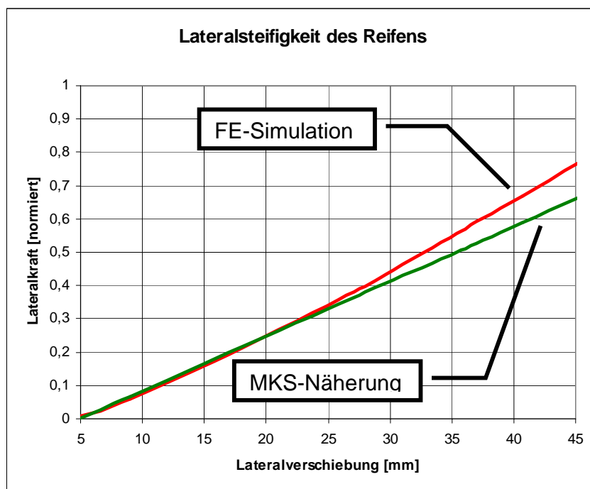
Bild 5: FE-Rechnung mit Kontakt (ABAQUS) zur Ermittlung der Lateralsteifigkeit
