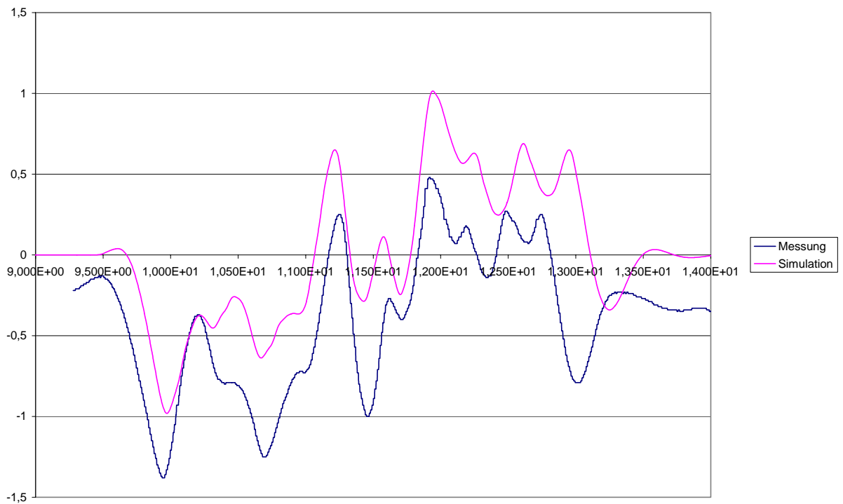
Bild 10: Vergleich Messung zu Simulation für den Nickwinkel (Offset nicht korrigiert).
