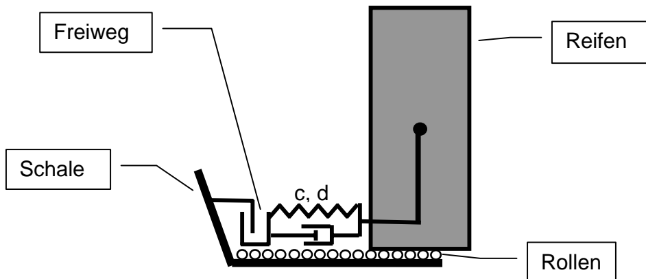
Bild 4: Reifen in Schale, Frontansicht
