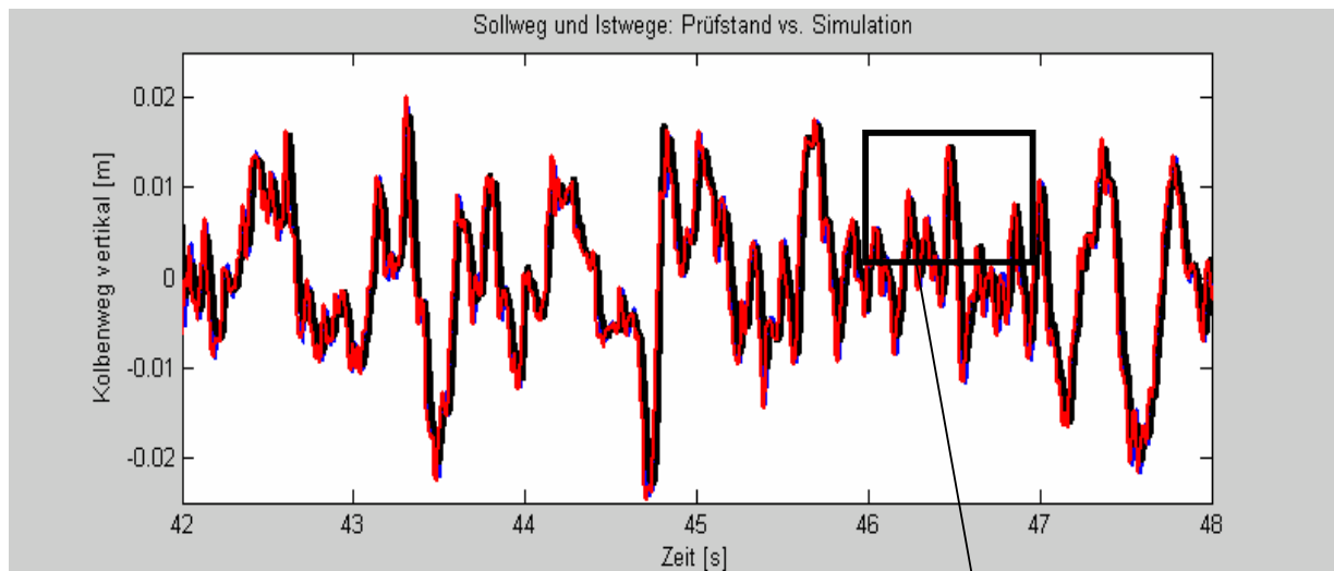
Bild 17: Vergleich Soll-Weg vertikal mit Ist-Weg gemessen am Prüfstand und aus Simulation (für Rauschsignal)
